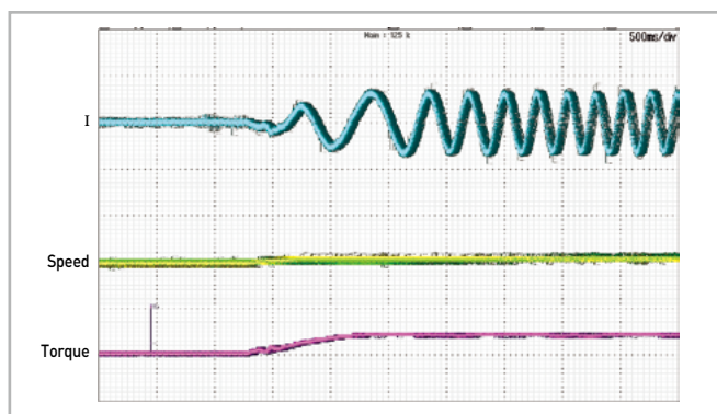
Krzywa startowa_2.2kW-4
