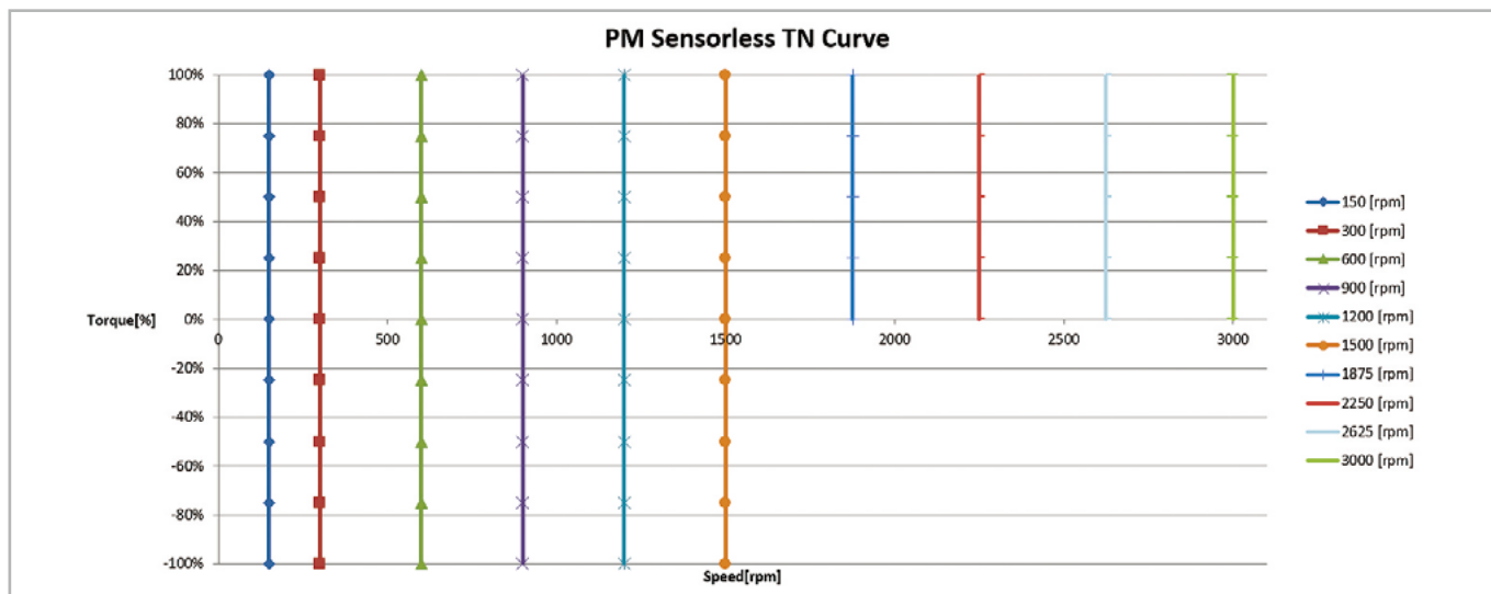
Krzywa dla_7.5kW-4
