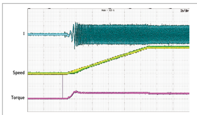
Krzywa startowa_2.2kW-4
