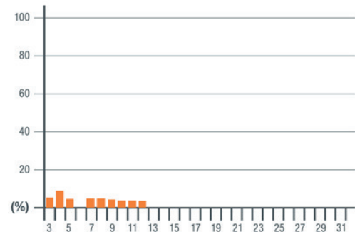
Armónicos con SINAF 3.0
