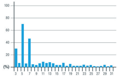
Armónicos sin SINAF 3.0
