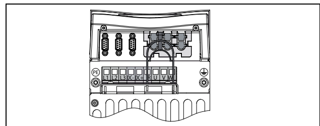
Rys. 11 Widok z dołu Emotron VFVFDU modele od 48-025 do 48-058 (rozmiar C2), z interfejsem kablowym do zasilania, silnika, DC+ / DC-, rezystorem hamowania i sterowaniem
