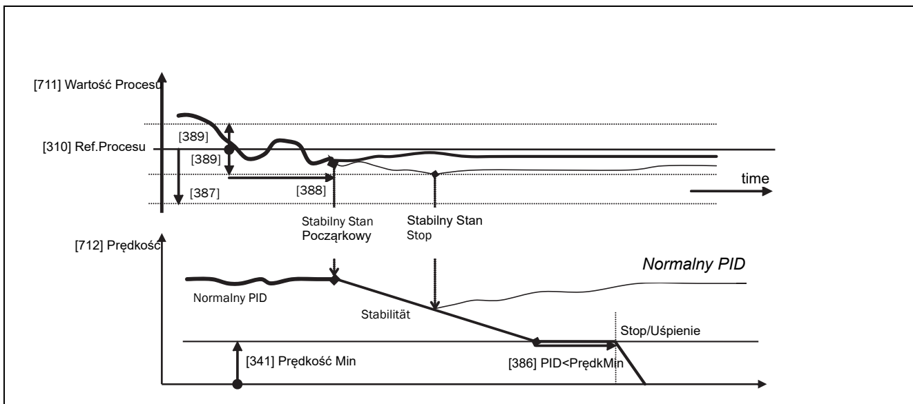
Rys. 98 Test stabilności
