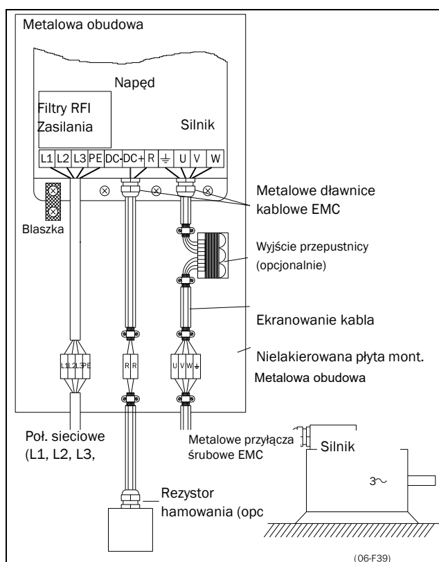
Rys. 37 Falownik na płycie montażowej w szafie sterowniczej
