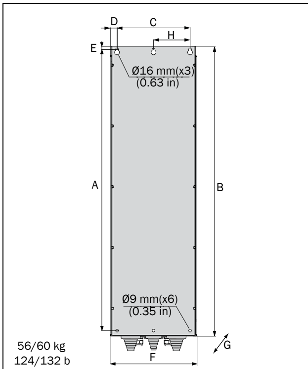
Fig. 16 Emotron VFXF DU Modele 48-090 do 175 (Rozmiar ramki E).
