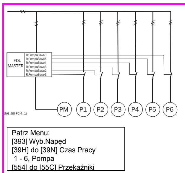
Rys. 68 Kontrola stałego MASTER
