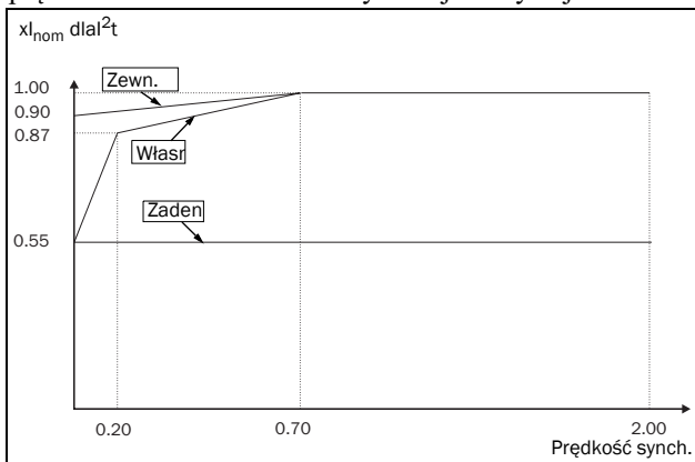
Rys. 78 I 2 t-Krzywa
