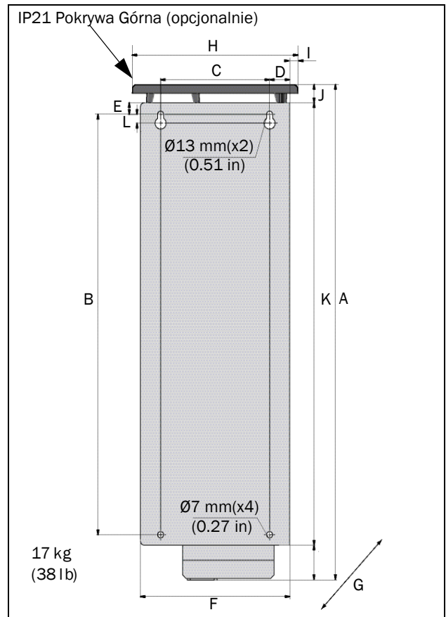
Rys. 10 Emotron VFVFDU Modele 48-025 do 48-058 (Rozmiar ramki C2), Widok z tyłu.
