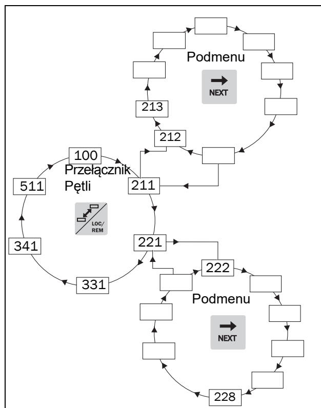
Rys. 72 Standardowy przełącznik pętli
