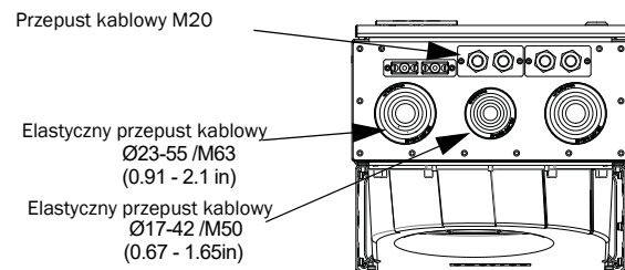
Fig. 18 Emotron VFXF DU Modele 48-210 do 295 (Rozmiar ramki F) Emotron VFXF DU Modele 69-90 do 200 (Rozmiar ramki F69).
