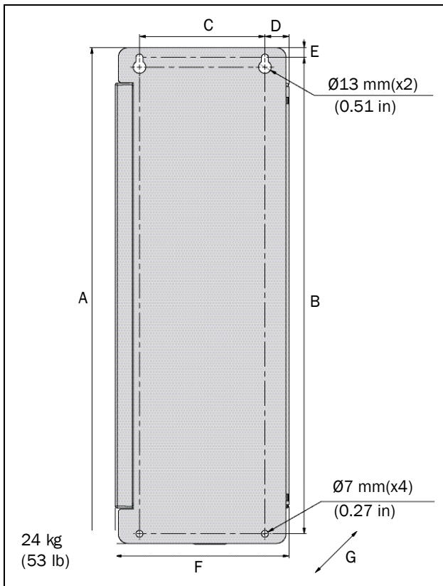
Rys. 8 Emotron VFVFDU Modele 48/52-026 do 046 (Rozmiar ramki C)
