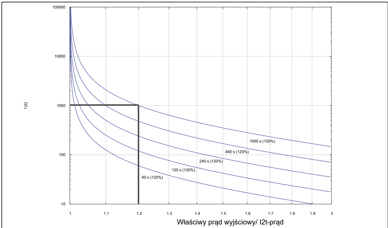
Rys. 79 Tryb I^2t
