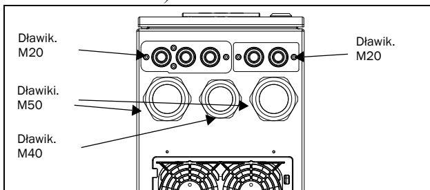
Rys. 12 Emotron VFDFU Modele 48/52-061 i 074 (Rozmiar ramki D)
