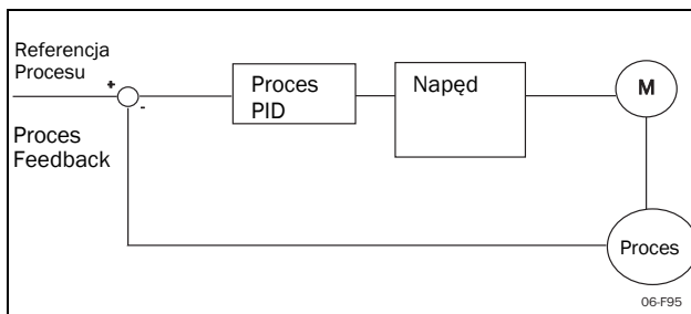
Rys. 95 Sterownik PID z zamkniętą pętlą
