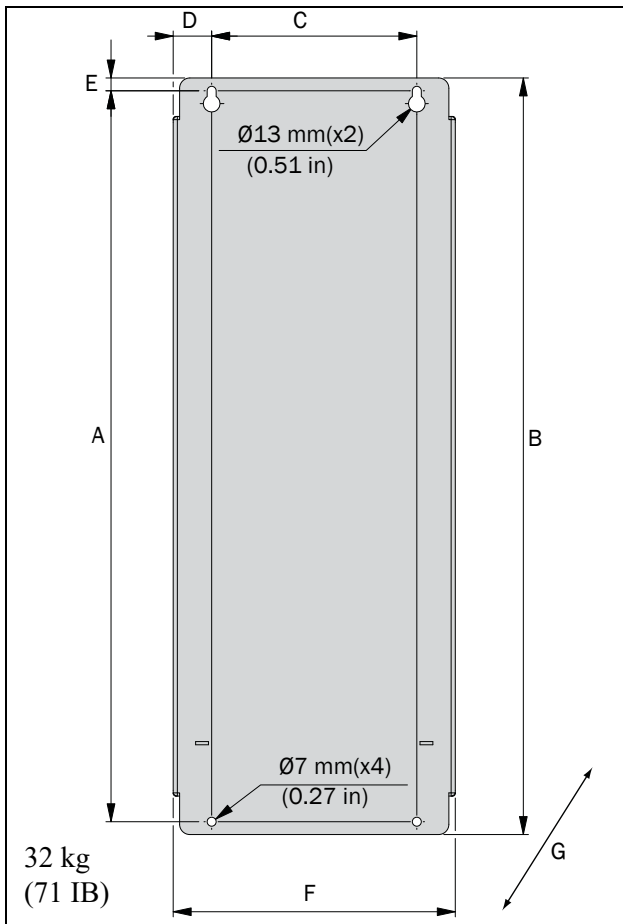
Rys. 12 Emotron VFDFU Modele 48/52-061 i 074 (Rozmiar ramki D)
