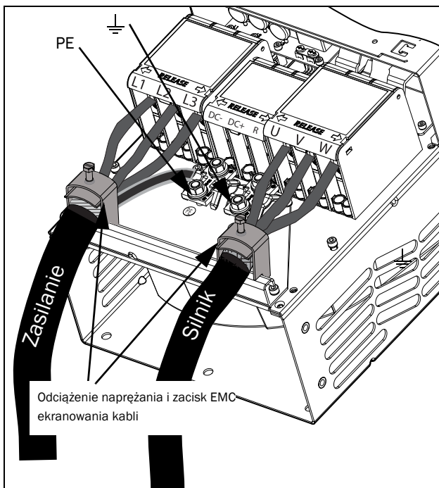
Rys. 34 Połączenia zasilania i silnika Modele 48-142 do 48-293 (rozmiary E2 i F2) z opcjonalnymi zaciskami dla DC, DC + i hamulca (rysunek zasadniczy)
