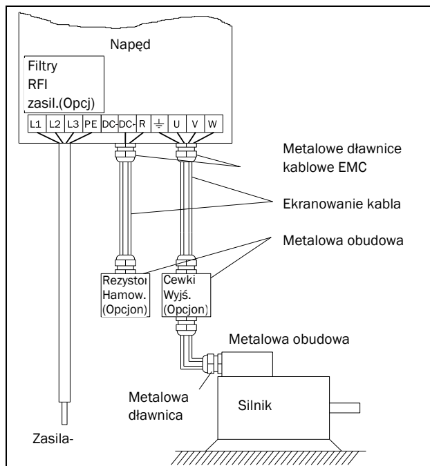
Rys. 54 Podłączenie przewodu sieciowego i silnika
