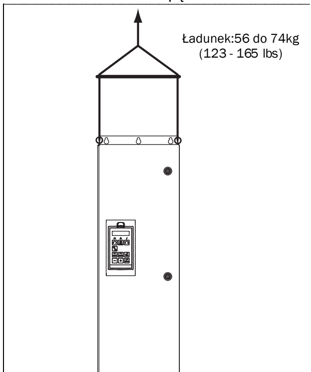
Rys. 2 Podnoszenie modeli napędów od -090 do -295
