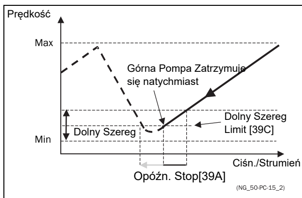
Rys. 102 Dolny szereg-limit
