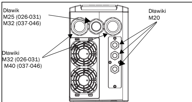
Rys. 9 Interfejs sieci, silnika i kabla komunikacyjnego, modele Emotron VFVFDU 48 / 52-026 do 046 (rozmiar C).
