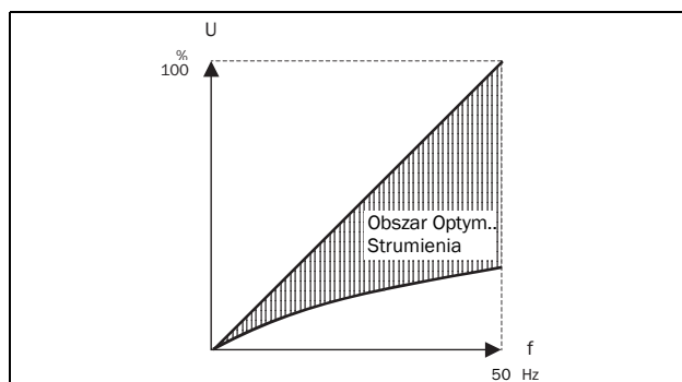
Rys. 93 Optymalizacja Strumienia
