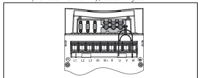
Rys. 15 Widok z dołu Model Emotron VFDFU 48-06072 do 48-105 (rozmiar ramki D2), z połączeniami kablowymi do sieci, silnika, DC+ / DC-, rezystorem hamującym i sterowaniem.
