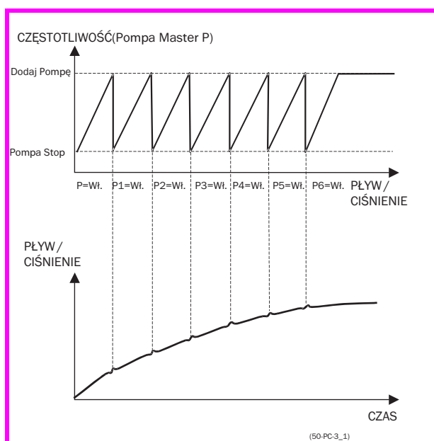
Rys. 67 Podstawowa zasada kontroli
